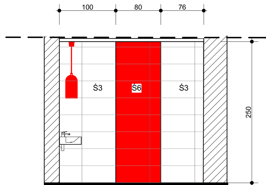
WIDOK ŚCIANY S4
