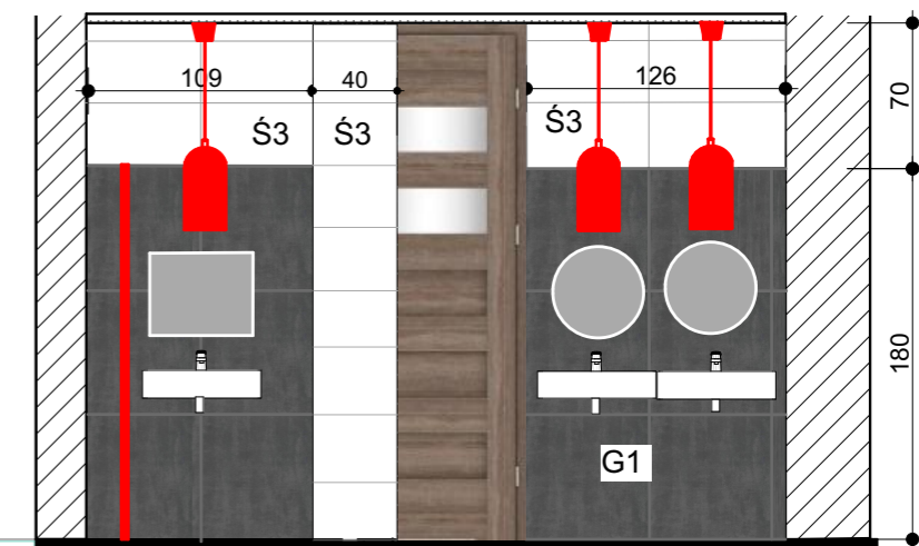
WIDOK ŚCIANY S3
