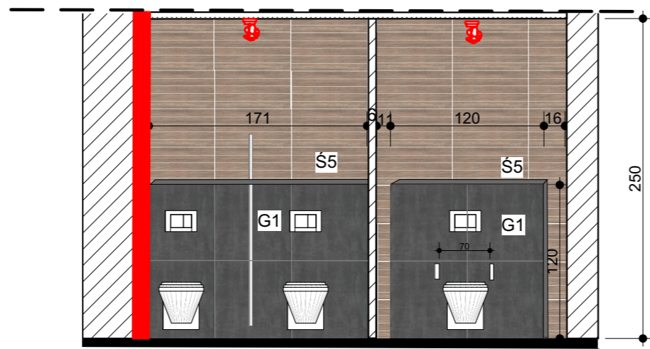
WIDOK ŚCIANA S2
