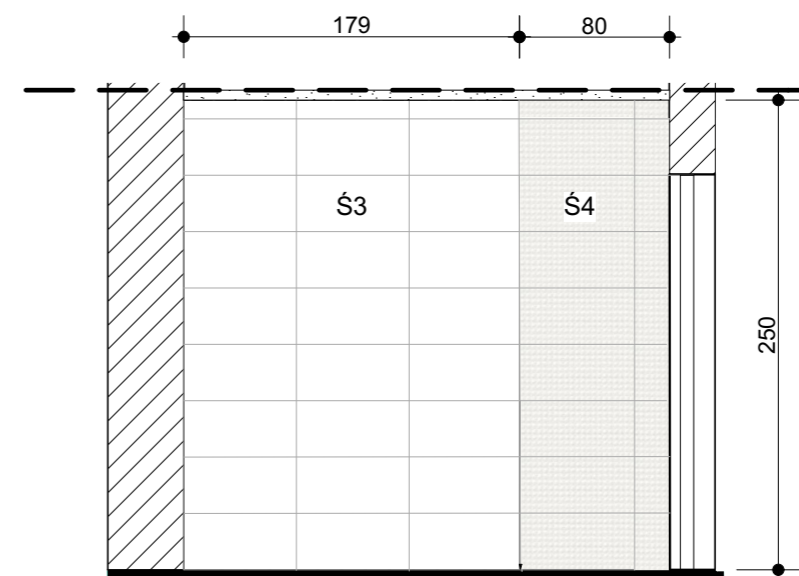
WIDOK ŚCIANY S5b
